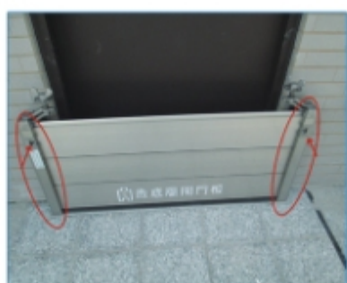
外牆安裝法
